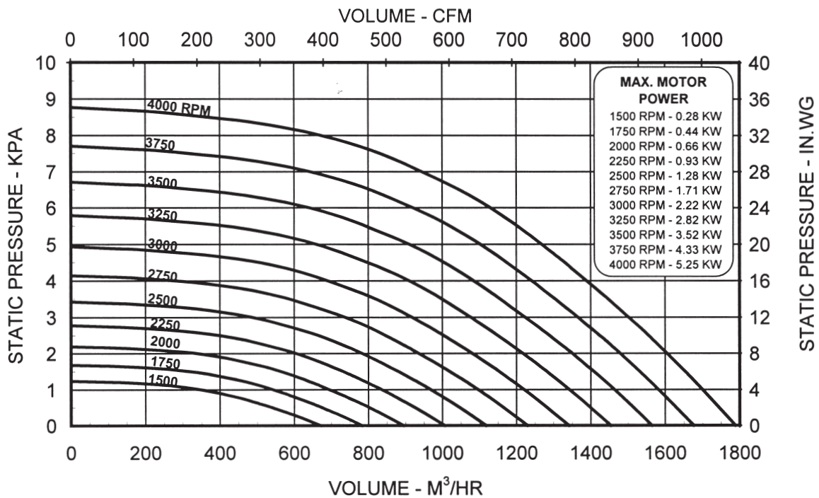
MODEL F24 FAN - BELT DRIVE
