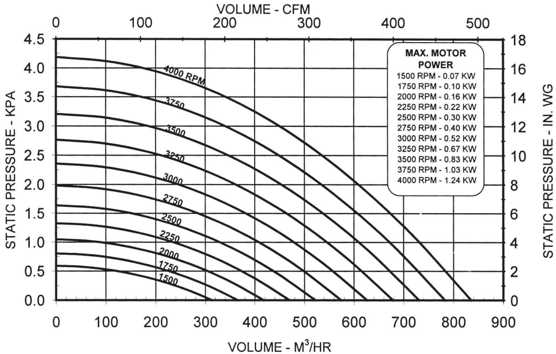
MODEL F10 FAN - BELT DRIVE
