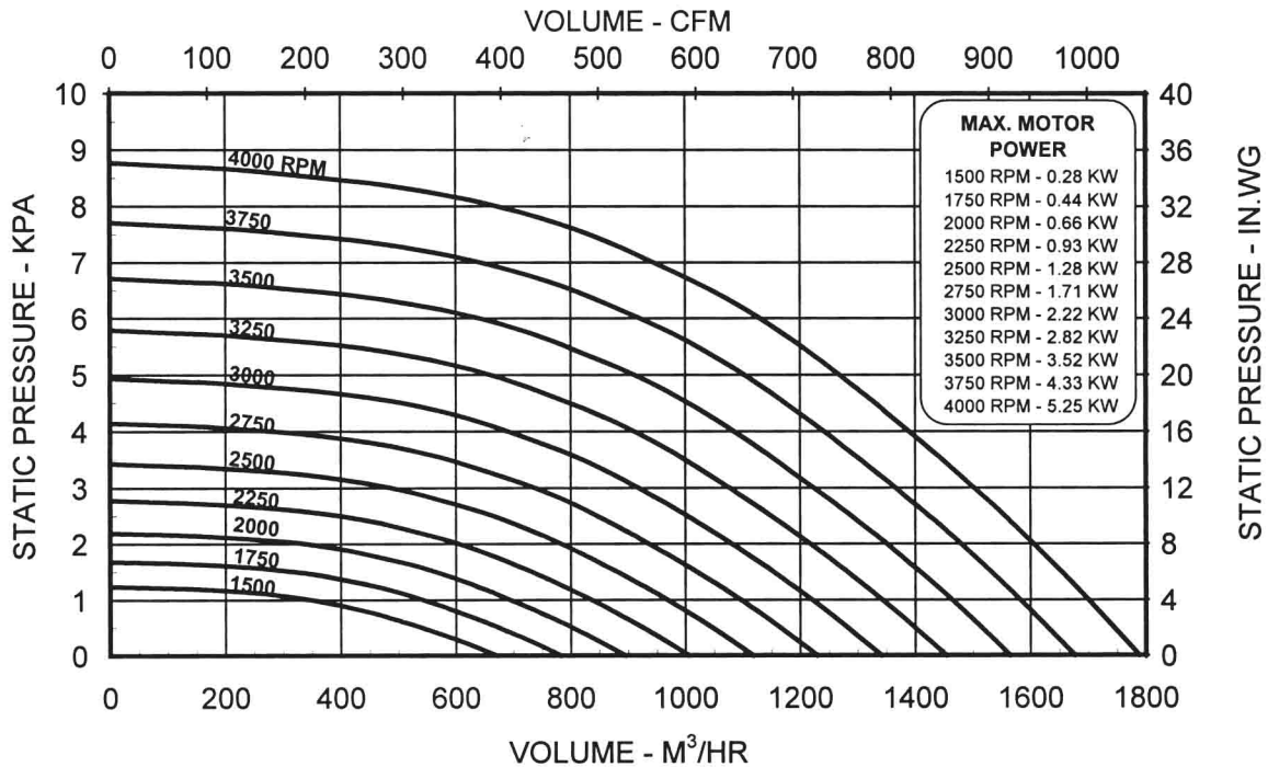
MODEL F24 FAN - BELT DRIVE
